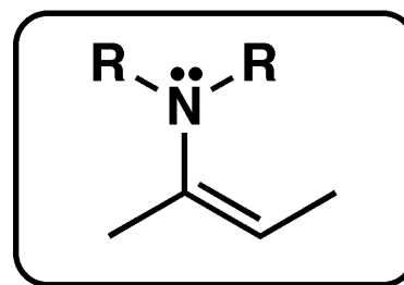
enamine
