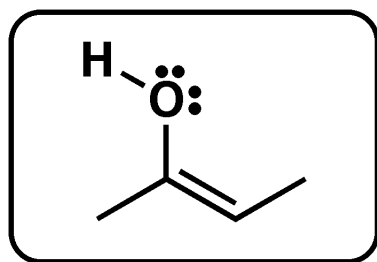
enol
